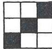
RAPPORT D'ARMURE 3 FILS - 3 DUITES
