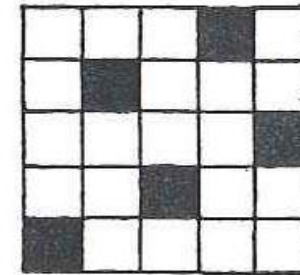
RAPPORT D'ARMURE 5 FILS - 5 DUITES
