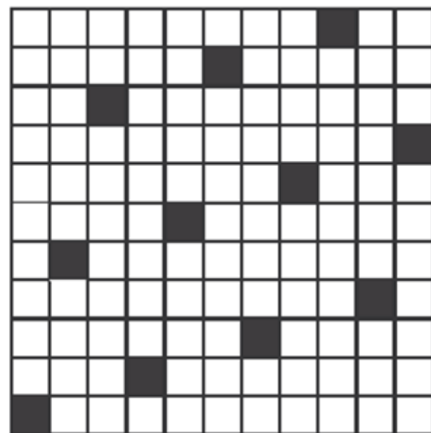
Figure 1 : Satin de module 11, décochement 4
